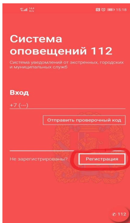
Рисунок 4. Выбор регистрации
