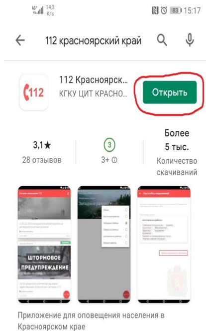
Рисунок 2. Запуск приложения
