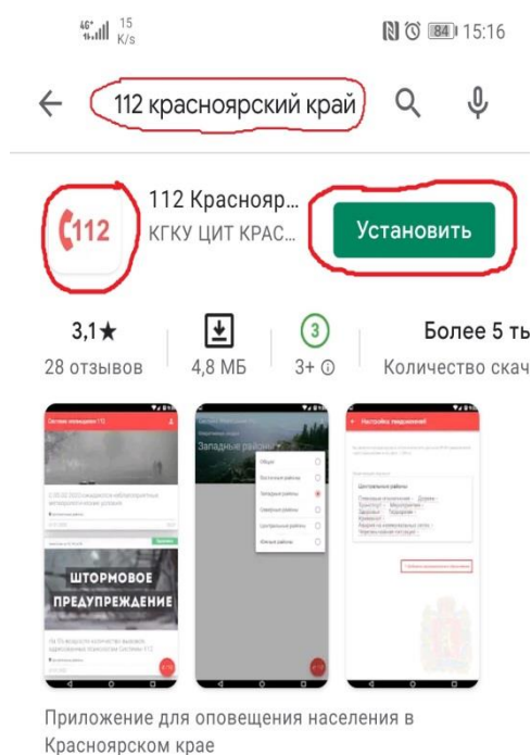
Рисунок 1. Установка приложения
